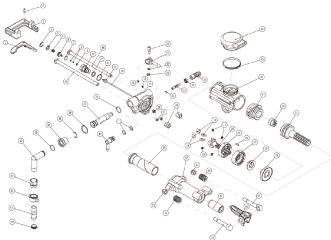
7655 气腿式凿岩机结构图
