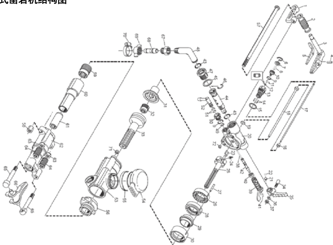
YT27 气腿式凿岩机结构图
