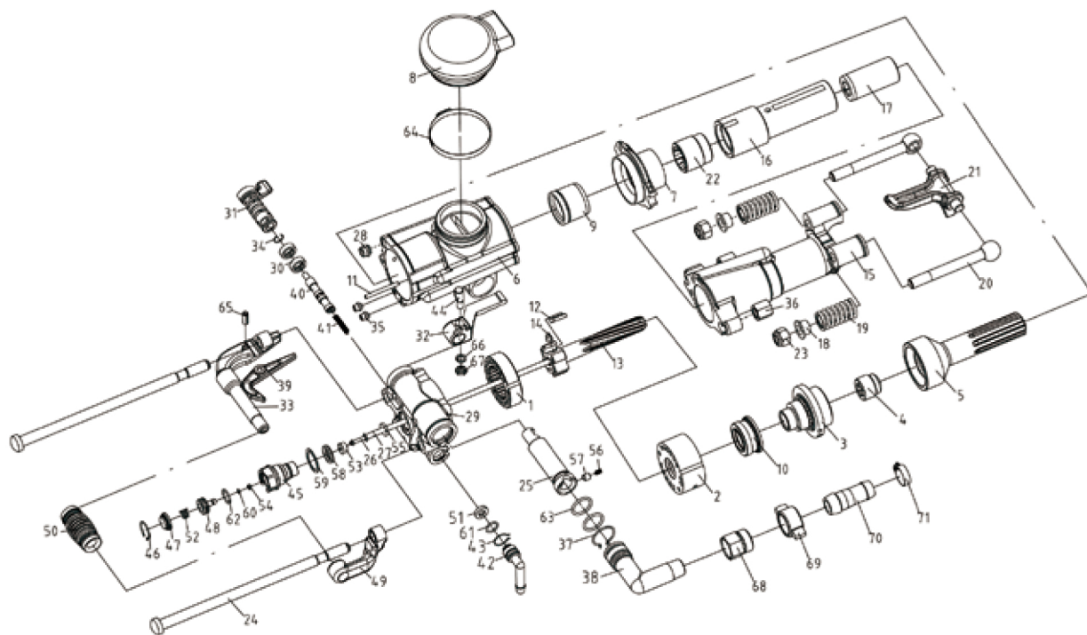
YT28气腿式凿岩机爆破图
