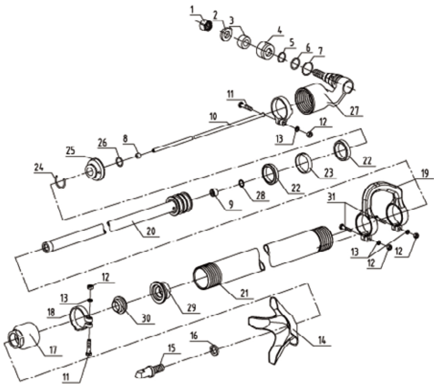
FT160A /FT160C 气腿结构图
